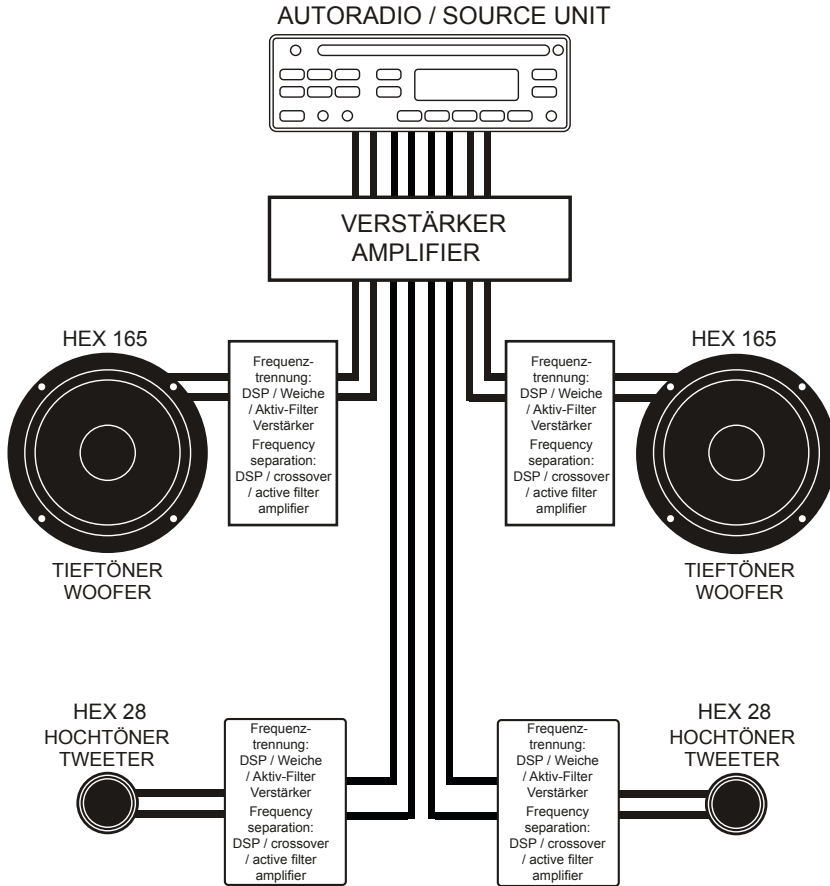
Anschlußplan für 2-Wege
